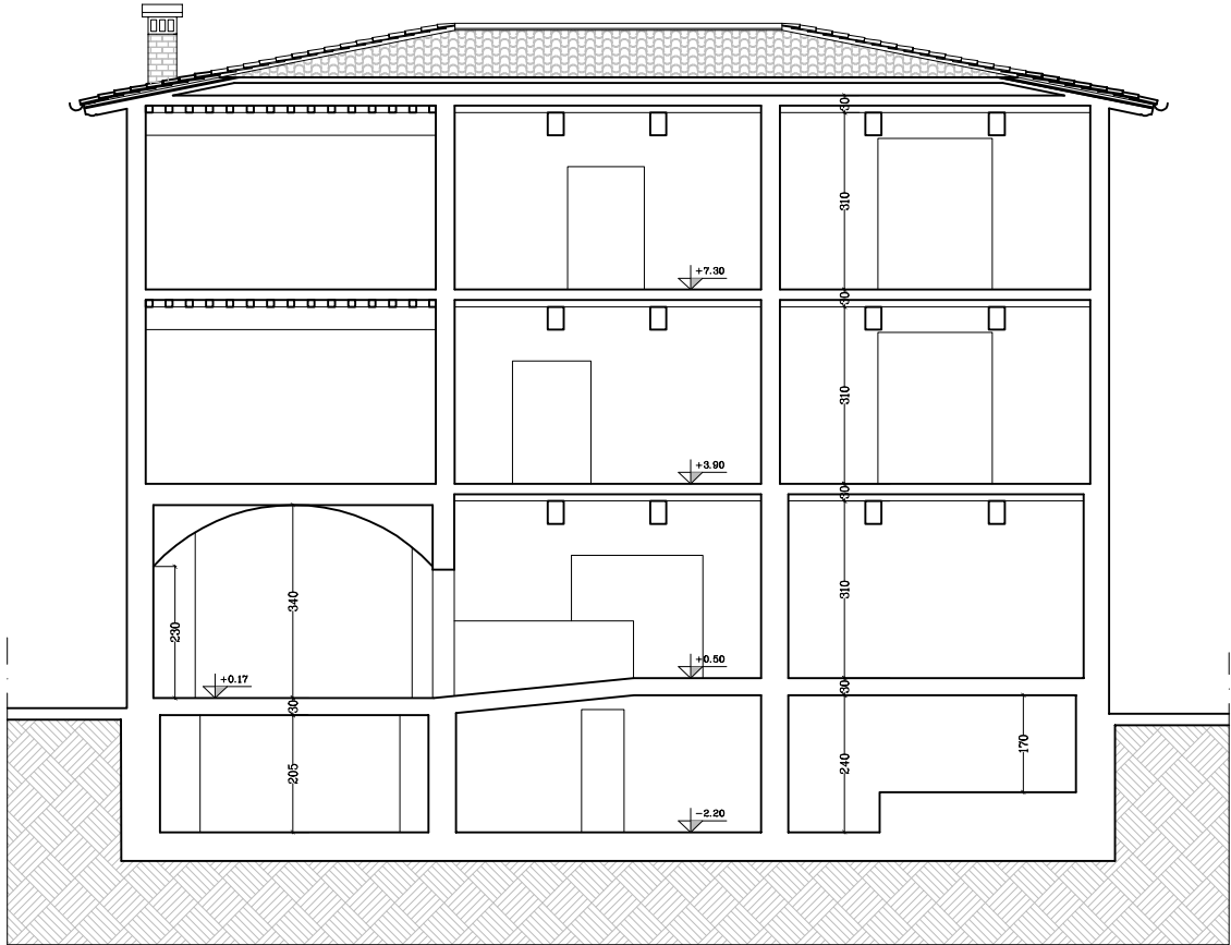
Sezione X - X'
