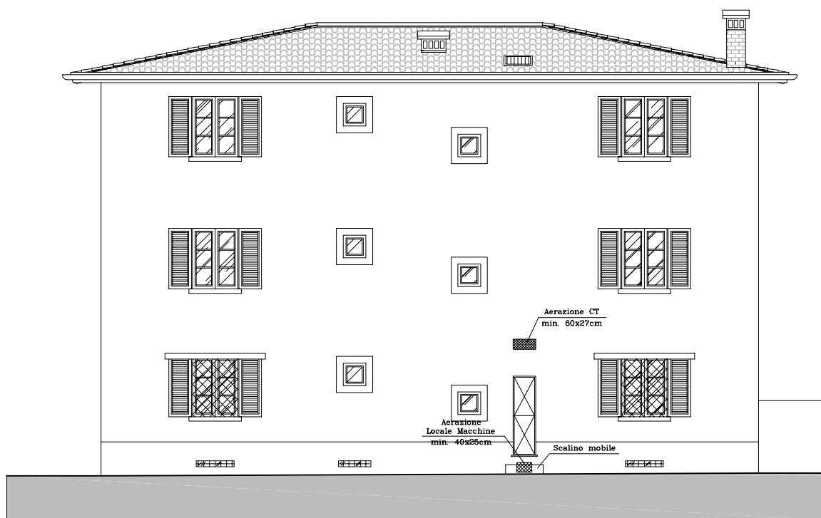
Prospetto Tergale
