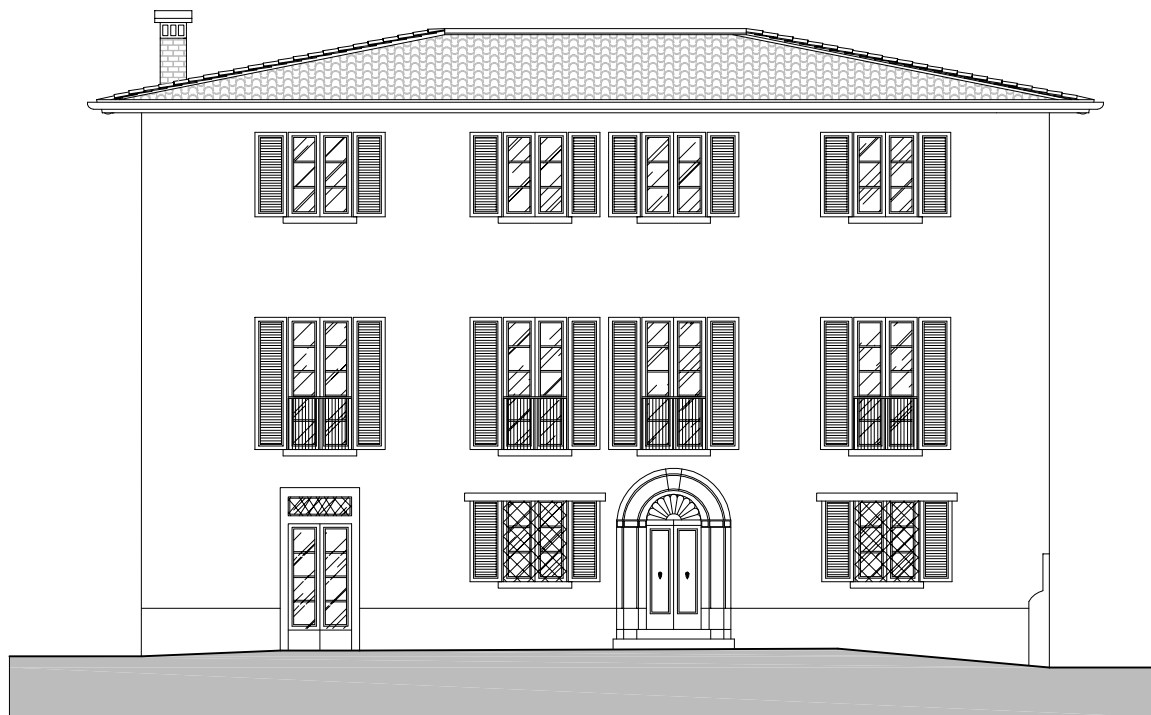
Prospetto Principale
