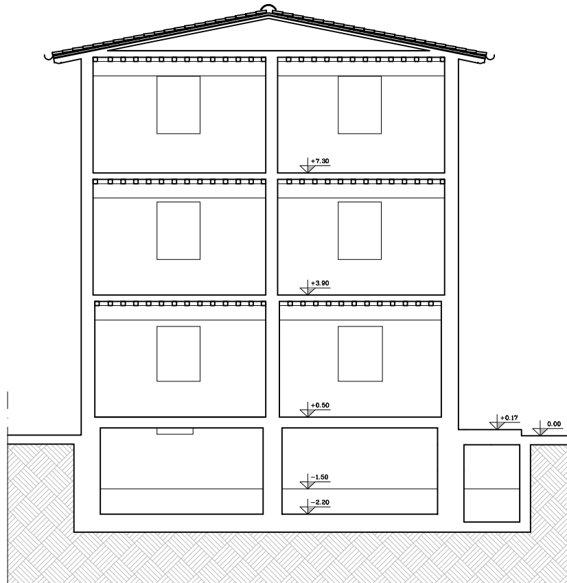
Sezione Y - Y'
