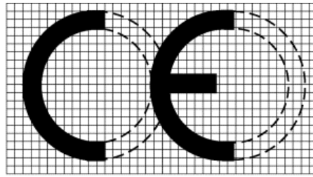
Figura 83.1 - Marchio CE
