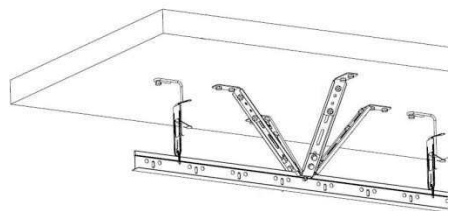
Esempio di controventamento antisismico
