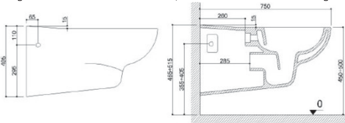
WC Rimless / Senza brida
