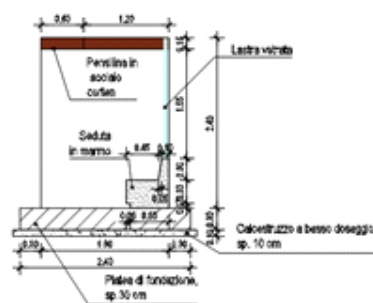
P2: PROSPETTO LATERALE Scala 1:50
