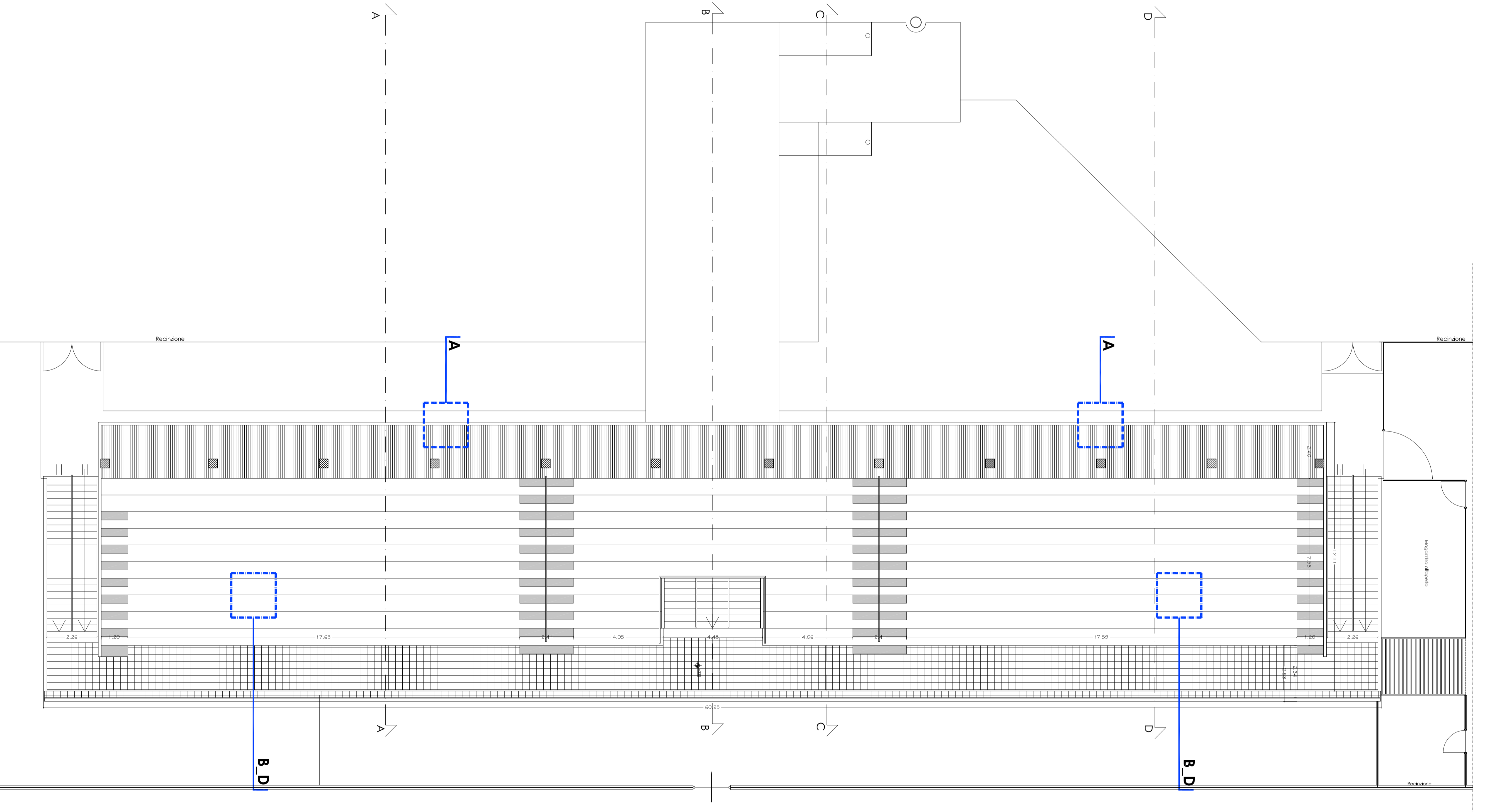
Pianta +335/+770
