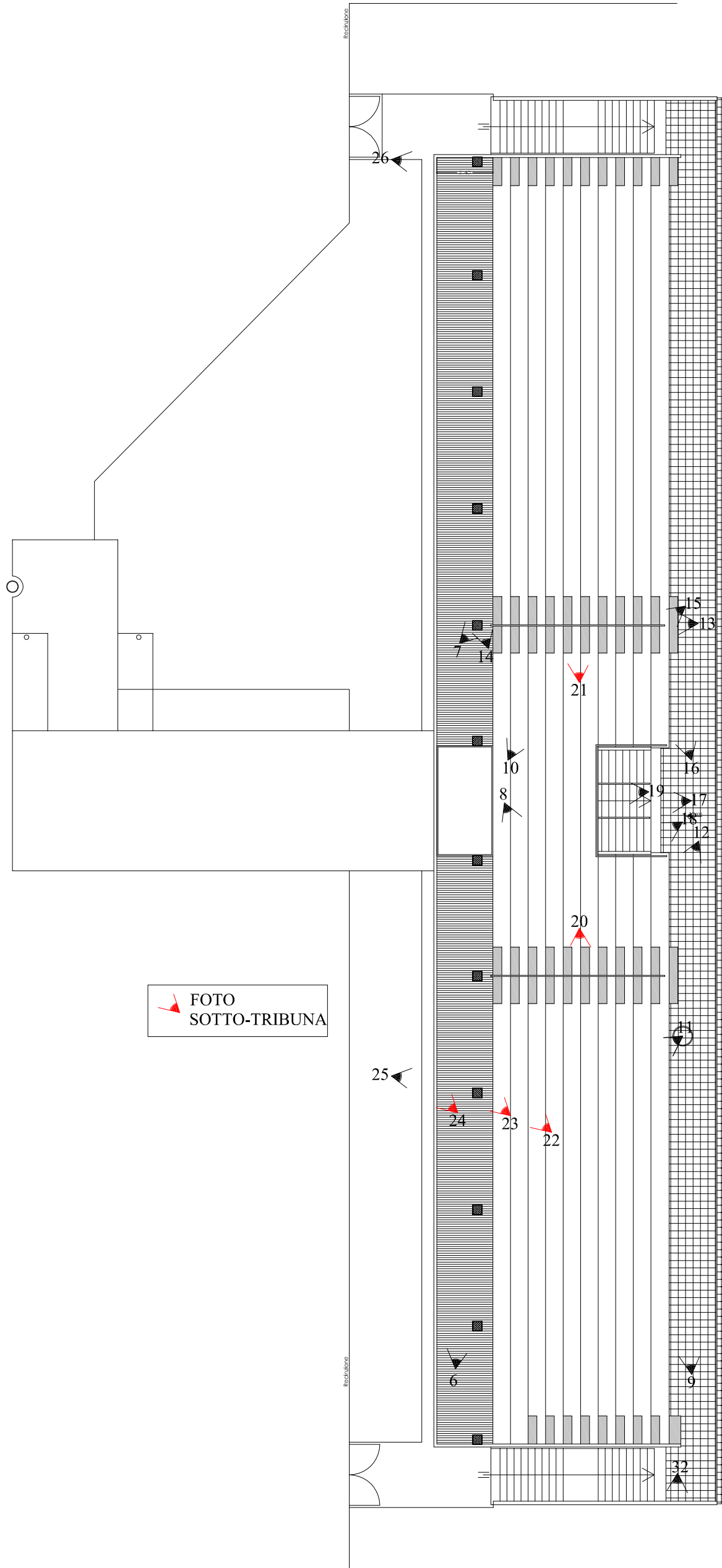
Pianta +335/+770
