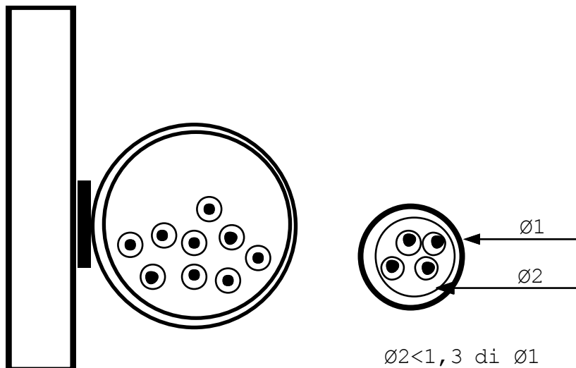
FIG. 1 )DIMENSIONAMENTO TUBAZIONI
