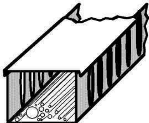
FIG.-3) INGRESSO CAVI NEI QUADRI _ DI IP 44- (particolare)
