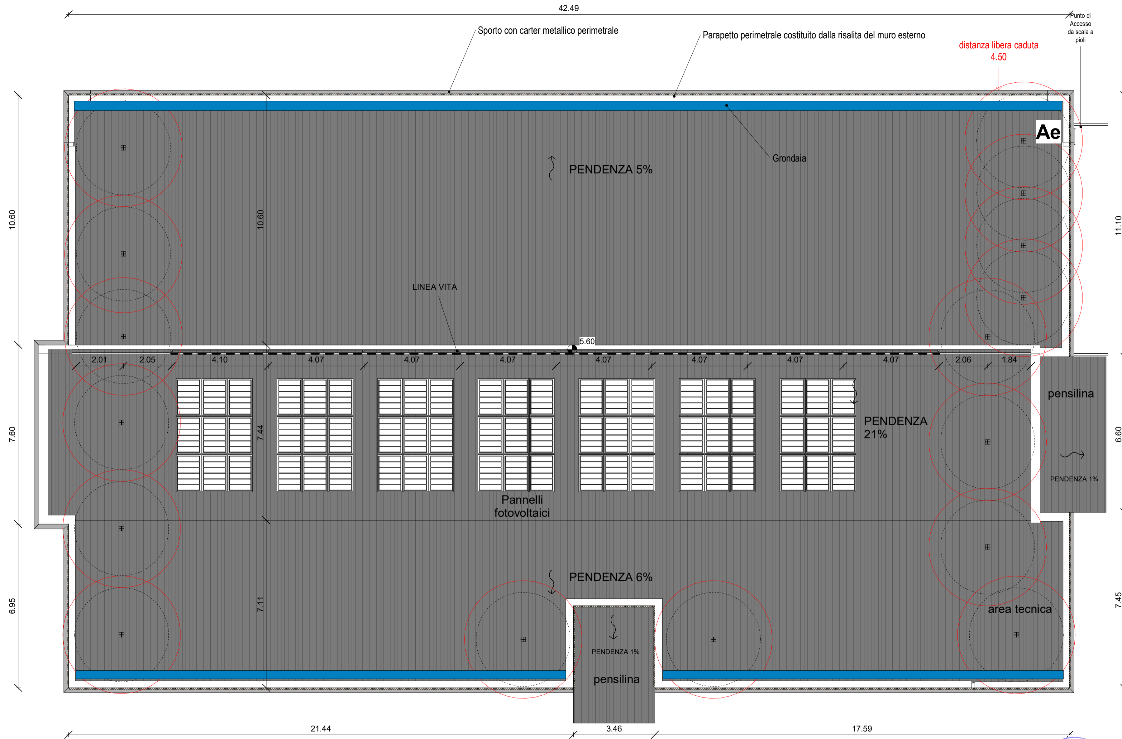
1 Piano Copertura 1:100
