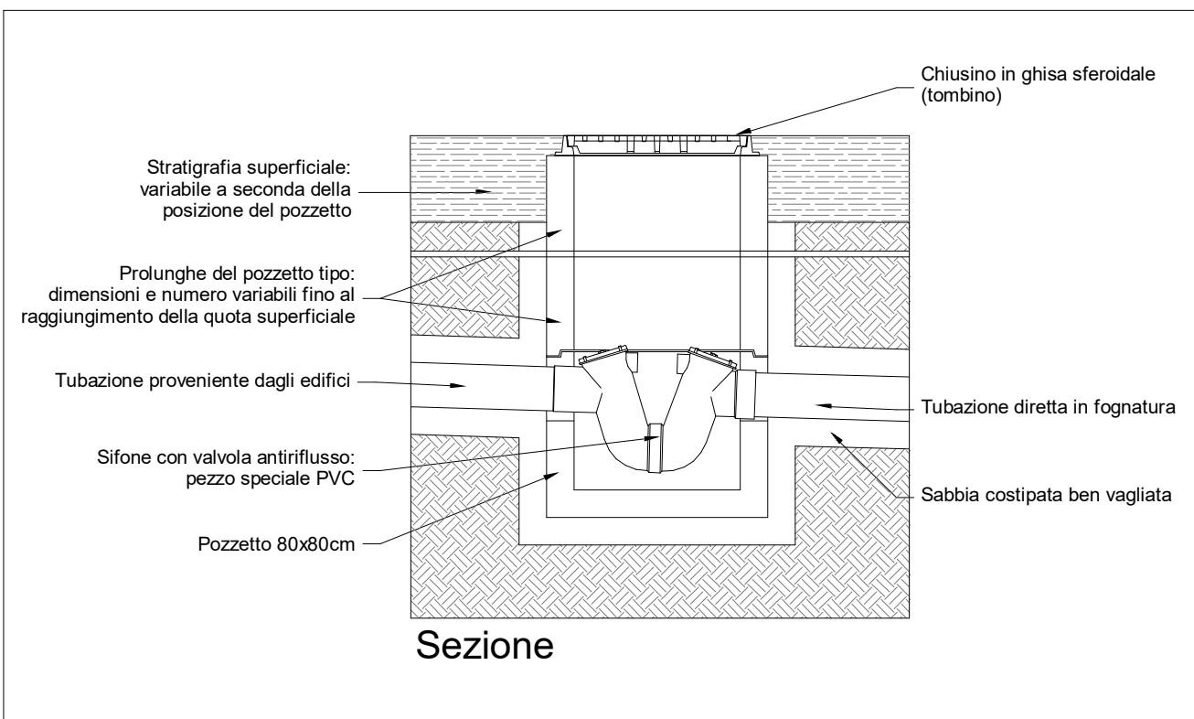
DETTAGLIO POZZETTO SIFONATO FOGNATURE ACQUE NERE - SCALA1:25
