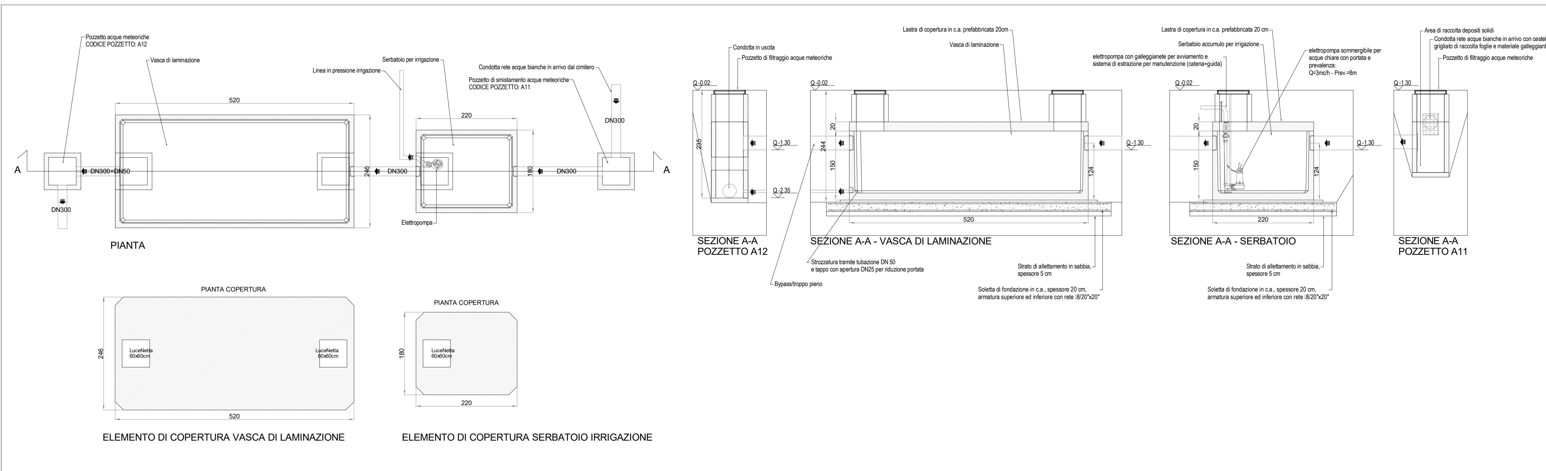
IMPIANTI PER ACQUE METEORICHE: SERBATOIO E VASCA DI LAMINAZIONE - SCALA 1:50
