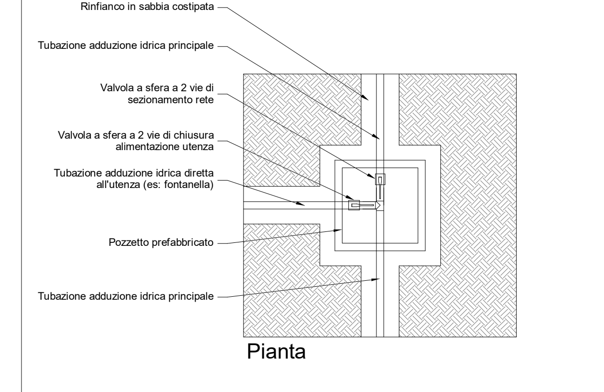
DETTAGLIO POZZETTO ADDUZIONE IDRICA FONTANELLE - SCALA1:25
