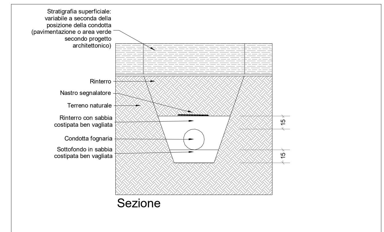
DETTAGLIO CONDOTTE FOGNARIE - SCALA1:25
