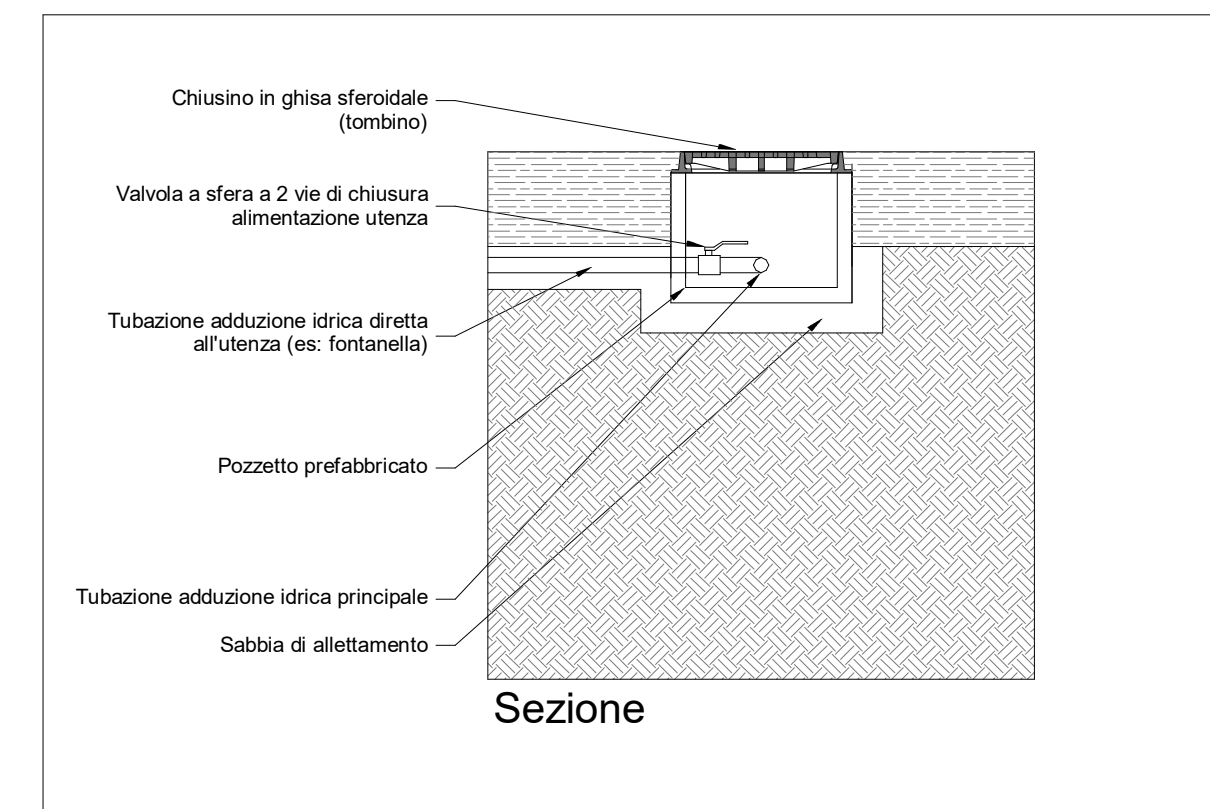
DETTAGLIO POZZETTO ADDUZIONE IDRICA FONTANELLE - SCALA1:25
