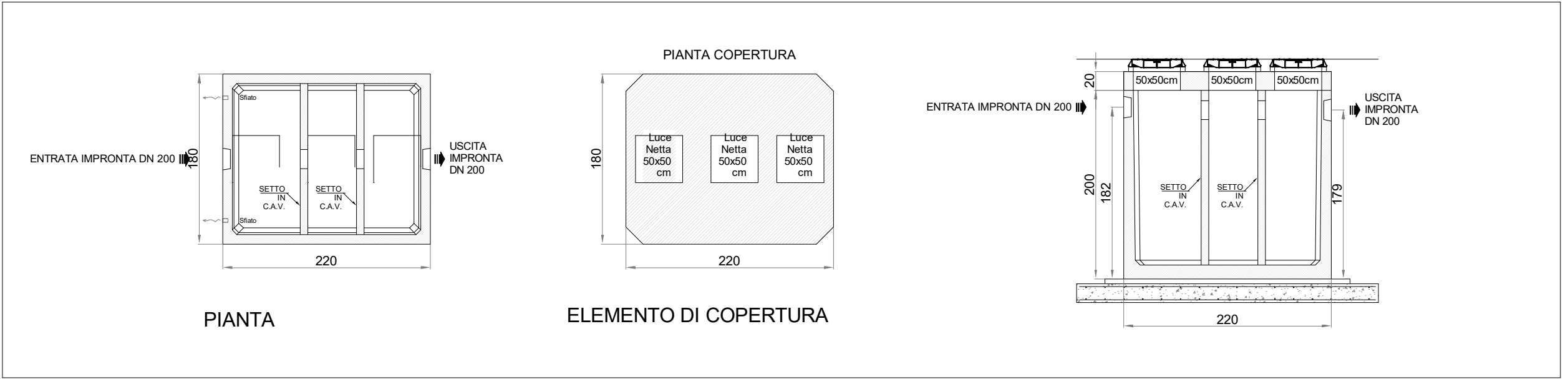
IMPIANTI PER ACQUE NERE: FOSSA SETTICA TRICAMERALE - SCALA 1:50
