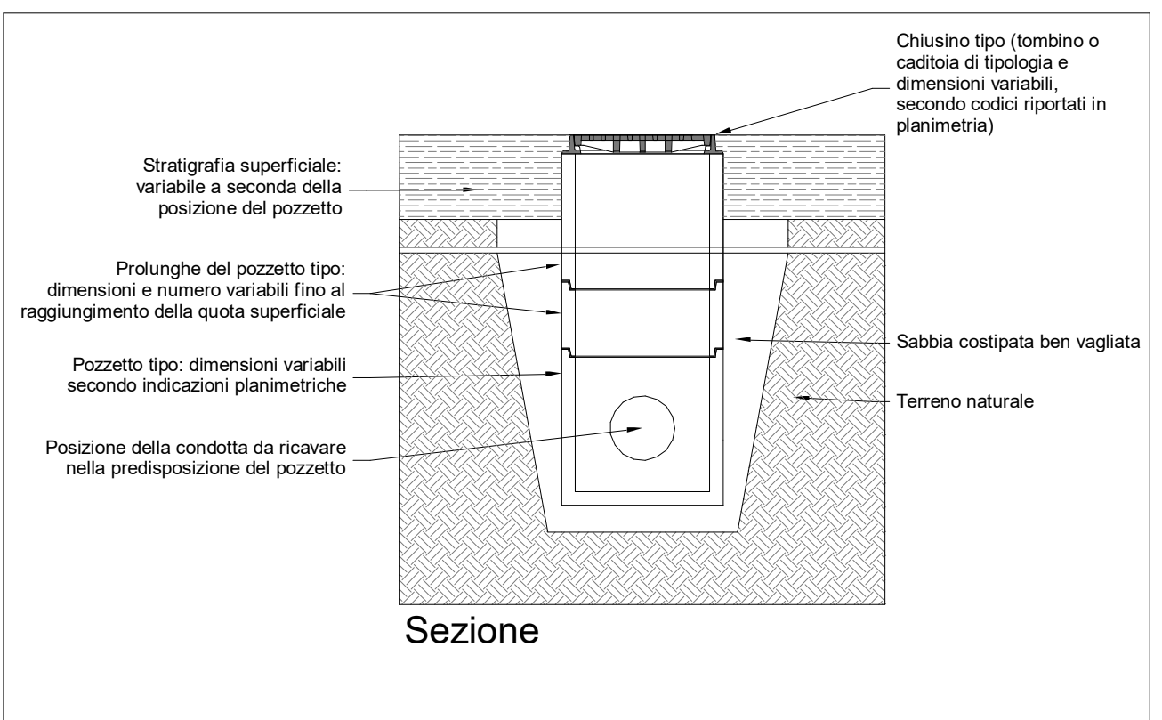
DETTAGLIO POZZETTO TIPO - SCALA1:25
